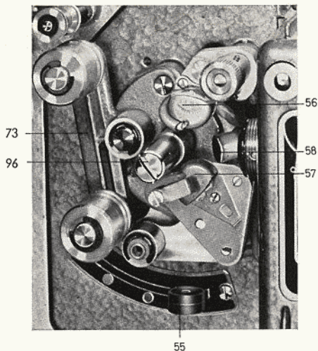
Bi d 30 Tongerät (Rotierende Tonbahn abgenommen)
