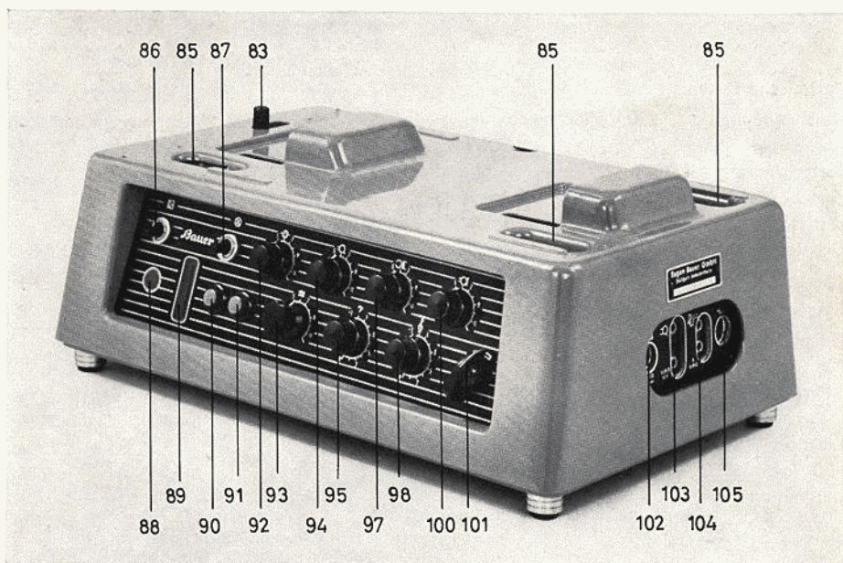
Bild 31 BAUER-15-W-Untersatzverstärker P V 5 M 1/3
