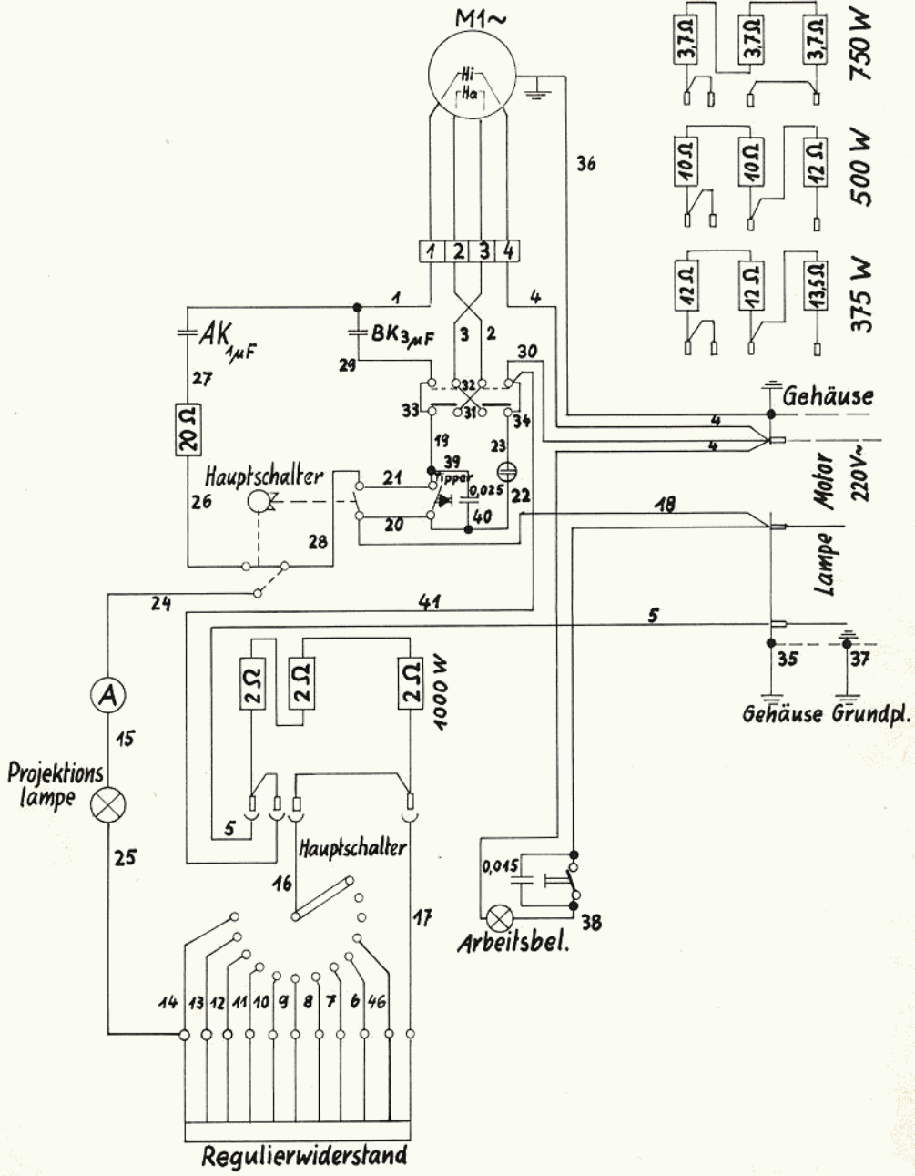
Bild 35 Schaltbild SS 768. BAUER-P 5-Stummprojektor mit Widerstandsbetrieb
