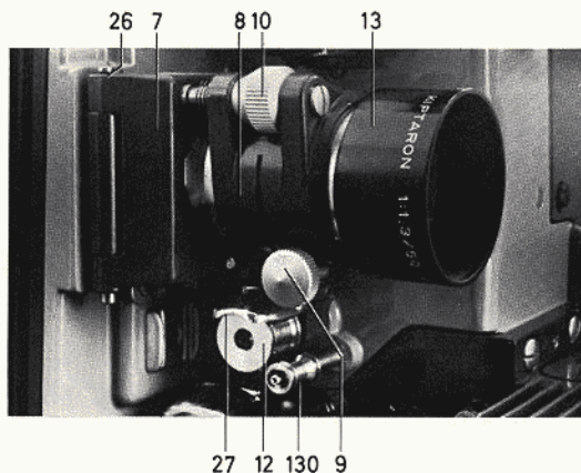
Bild 26 Objektivhalter
