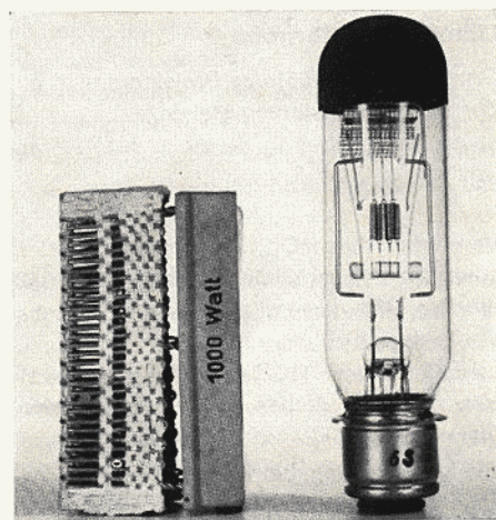
Bild 15 Projektionslampe 1000 W/100 V mit Einsteckwiderstand
