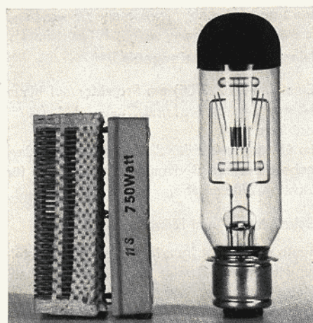
Bild 14 Projektionslampe 750 W/100 V mit Einsteckwiderstand
