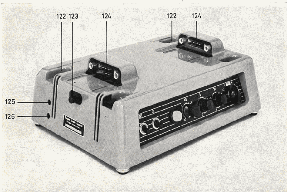
Bild 34 BAUER-6-Watt-Untersatzverstärker PV 5 T 3/1
