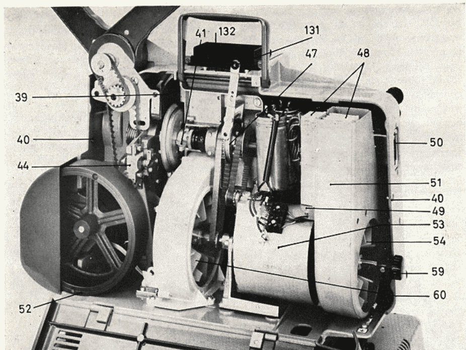
Bild 17 Innenansicht des BAUER-P 5-Tonprojektors. Gehäusedeckel offen.
