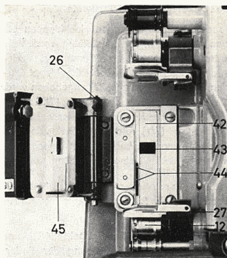
Bild 23 Filmtür
