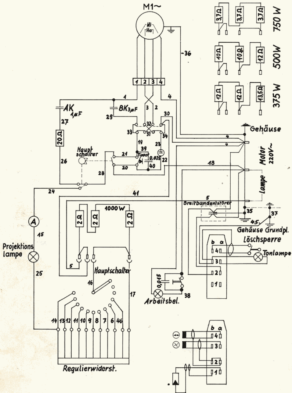
Bild 36 Schaltbild SS 765. BAUER-P 5-Tonprojektor mit Widerstandsbetrieb
