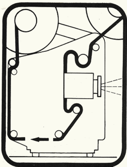
Bild 8 Filmeinlegschemata für den Stummprojektor
