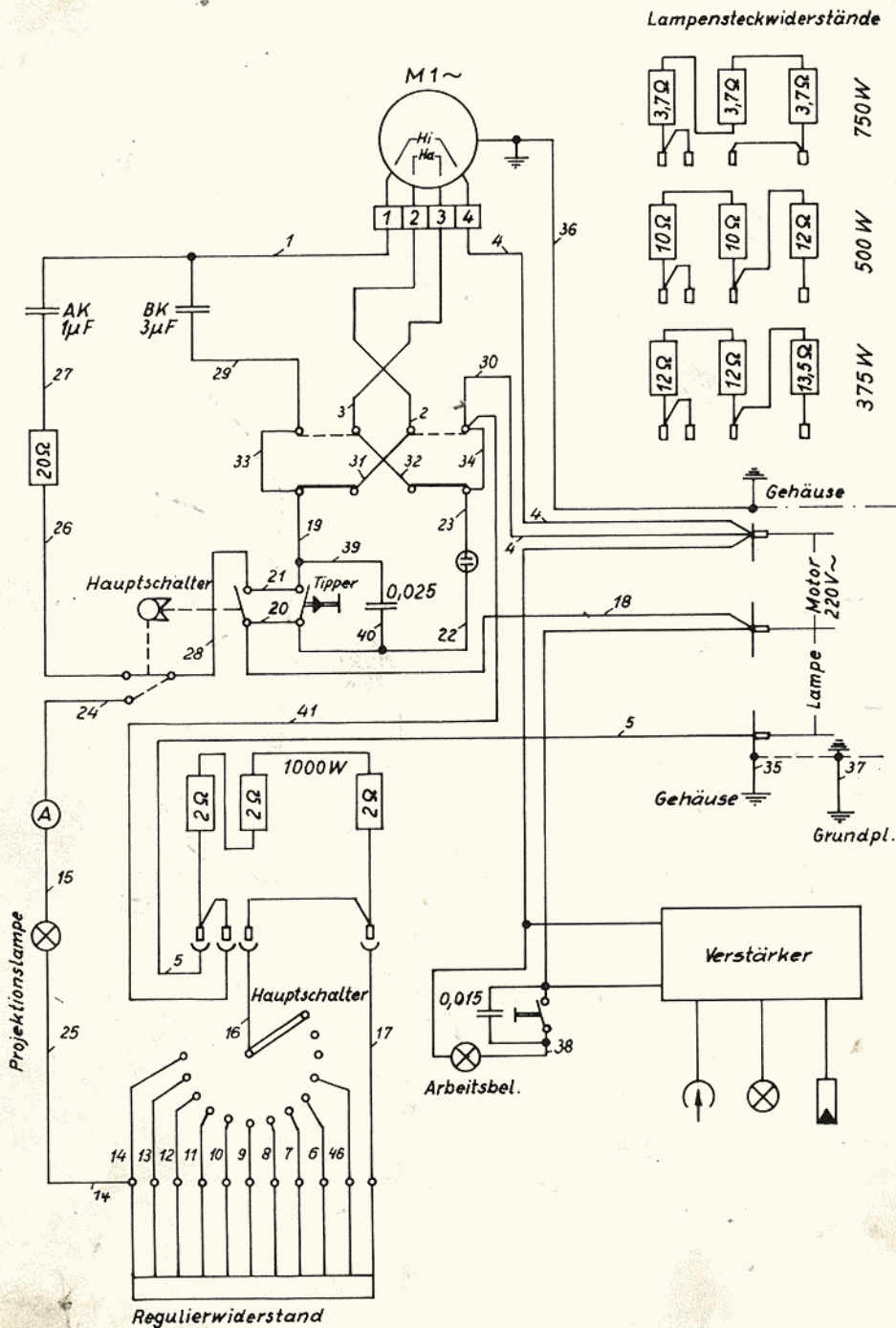
Bild 38 Schaltbild SS 765 b BAUER-P 5 mit Widerstandsbetrieb und eingebautem Transistor-Verstärker
