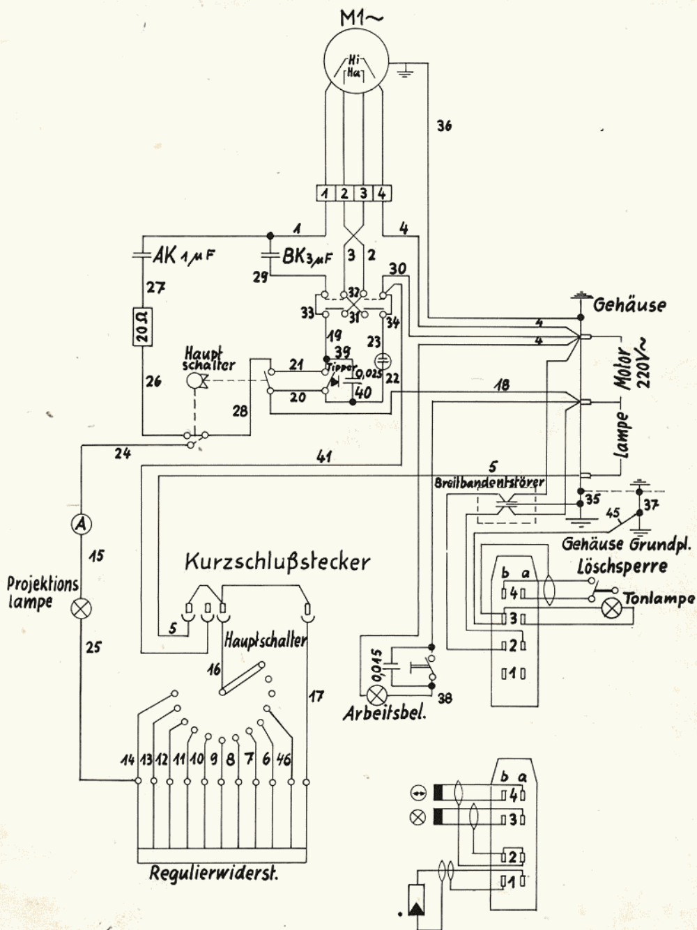
Bild 37 Schaltbild SS 767. BAUER-P 5-Tonprojektor mit Transformatorbetrieb
