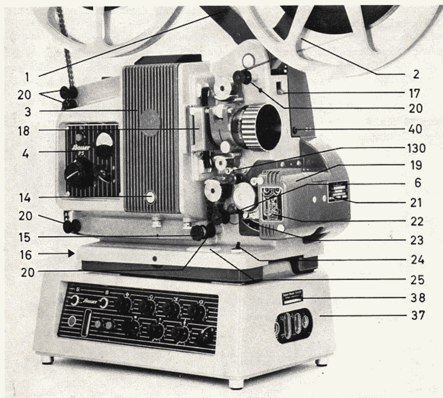
Bild 7 BAUER-P 5 M 15-Tonfilmprojektor mit 15-W-Untersatzverstärker
