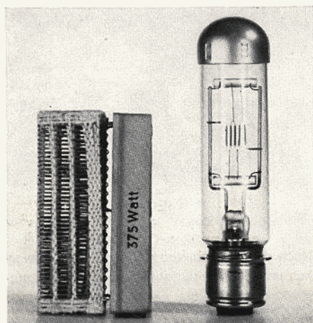
Bild 12 Projektionslampe 375 W/75 V mit Einsteckwiderstand
