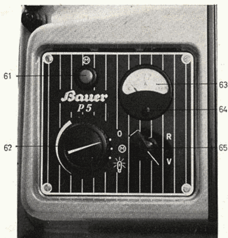
Bild 18 Schalterplatte
