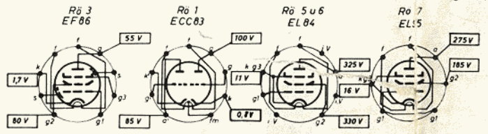
Bild 43 Schaltbild SS 746. BAUER-15-Watt-Untersatzverstärker PV5 T1/3
