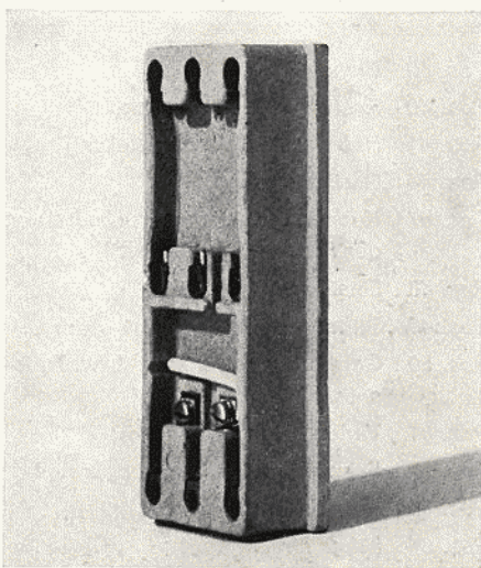
Bild 16b Kurzschlußstecker für Transformatorbetrieb
