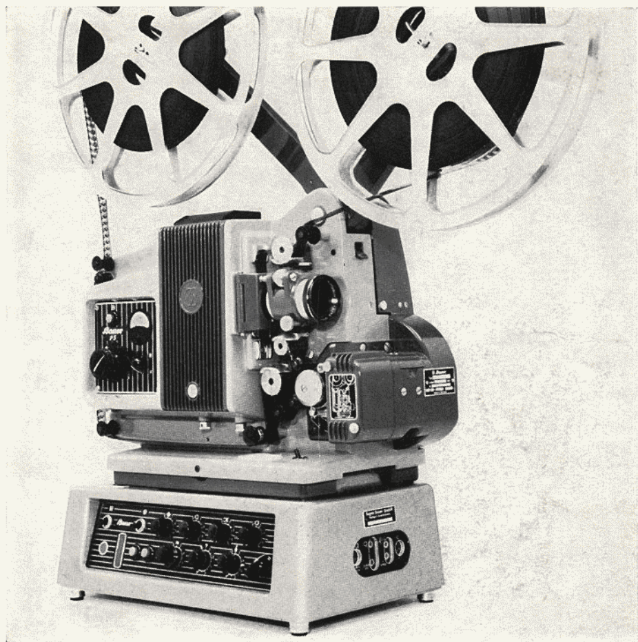
Bild 2 BAUER-P 5 M 15-Tonfilmprojektor P W 5 M 16 G 1 mit 15-W-Untersatzverstärker
