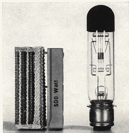
Bild 13 Projektionslampe 500 W/100 V mit Einsteckwiderstand
