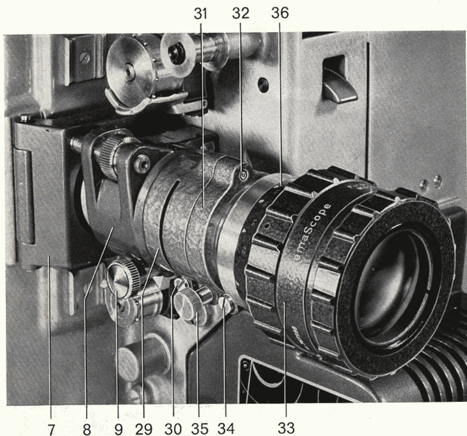
Bild 28 Objektivhalter mit Anamorphot (Schnellwechselfassung)
