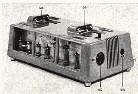
Bild 32 BAUER-15-W-Untersatzverstärker P V 5 M 1/3 (Schutzklappen abgenommen)
