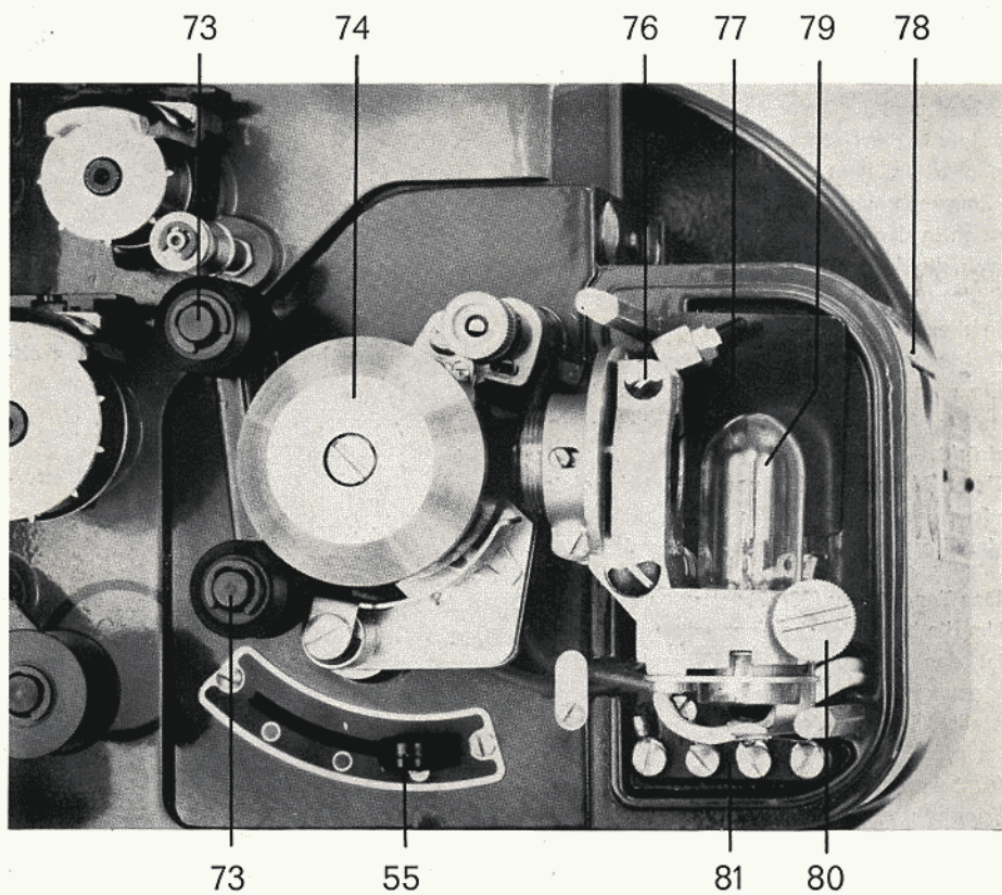
Bild 29 Tongerät (Schutzdeckel abgenommen)
