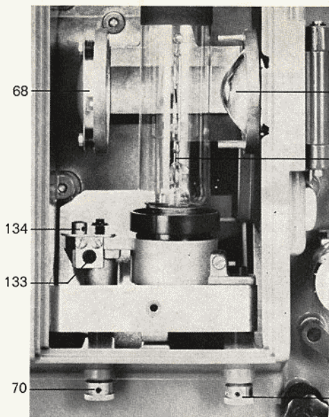
Bild 20 Lampenhaus, geöffnet
