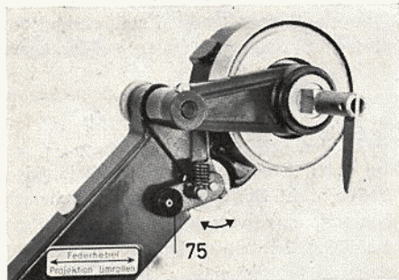
Bild 25 Friktion am vorderen Spulenarm
