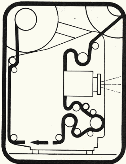
Bild 9 Filmeinlegschemata für den Tonprojektor
