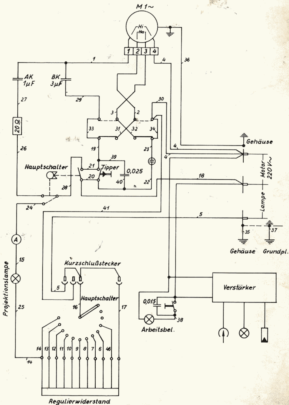
Bild 39 Schaltbild SS 767 c. BAUER-P 5 mit Trafobetrieb und eingebautem Transistor-Verstärker
