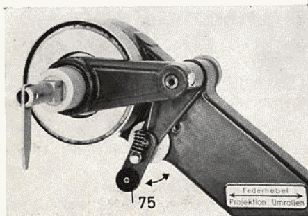
Bild 24 Friktion am hinteren Spulenarm
