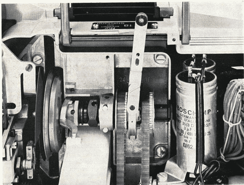
Bild 22 Blendenwelle mit Kupplungscheibe
