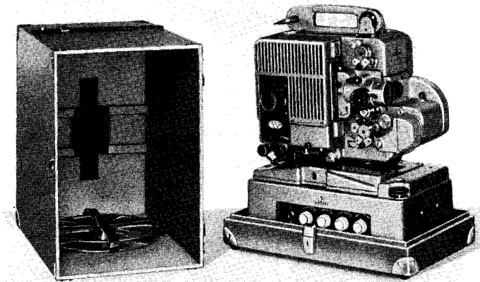
Bild 24 Projektor mit Lichttongerät und Verstärker auf Tragkofferboden, Kofferdeckel nebenstehend
