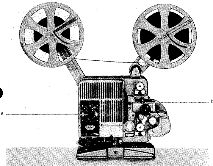
Bild 23 Umspulanordnung
