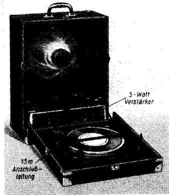
b Rückansicht – geöffnet
